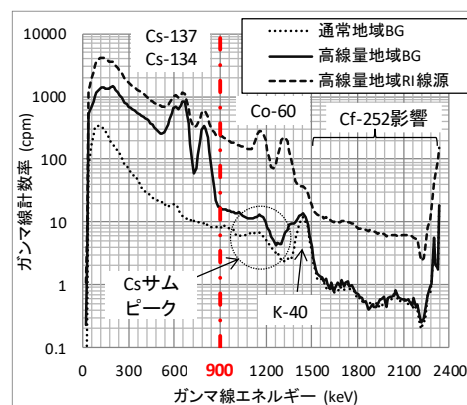
図-1 エネルギースペクトル測定結果
