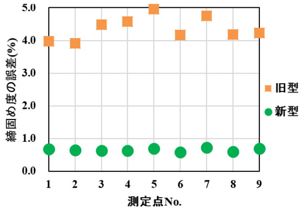
図 4 BG 測定点 1 ケ所で生じる締固め度の誤差
